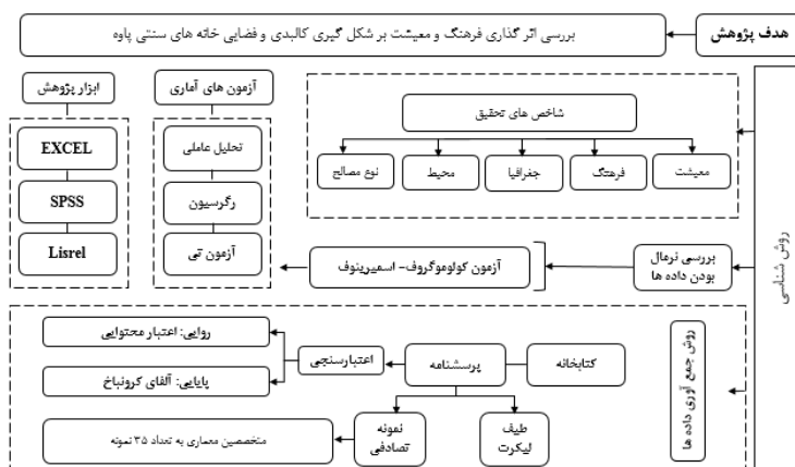
شکل ۱. روش‌شناسی تحقیق
