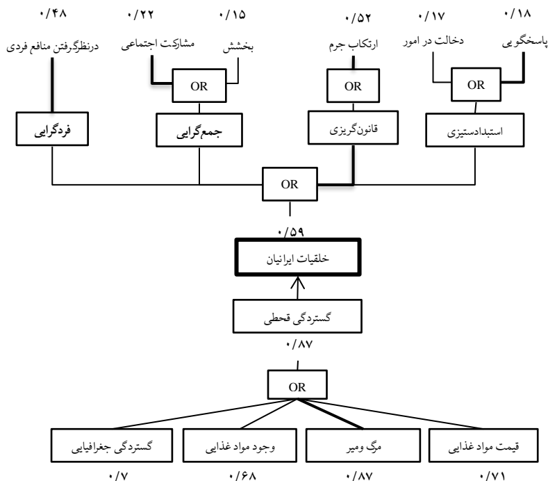
نمودار ۱. کالیبراسیون خلیقات ایرانیان در قحطی جنگ جهانی اول
